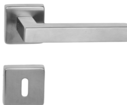
/// készleten CUBIC F szálcsiszolt acél A rozsdamentes acél M A=130 mm D=50x50 mm
