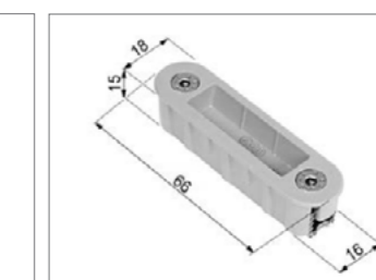
Alutop XT megfordítható zárólemez fém tokhoz
