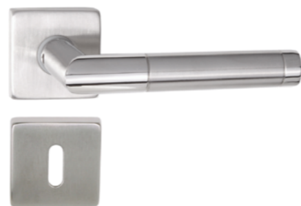
/// készleten PANAMA négyzetözöttás F fényes és szálcsiszolt acél A rozsdamentes acél M A=130 mm D=50 mm
